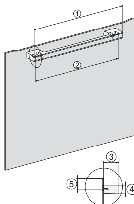
Seitenansicht H7000 M, Skizze, GB, AU
